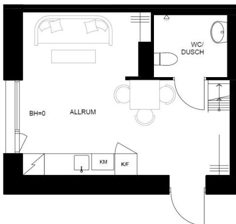
NEDRE PLAN
