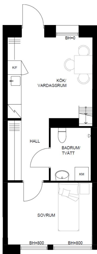
NEDRE PLAN
