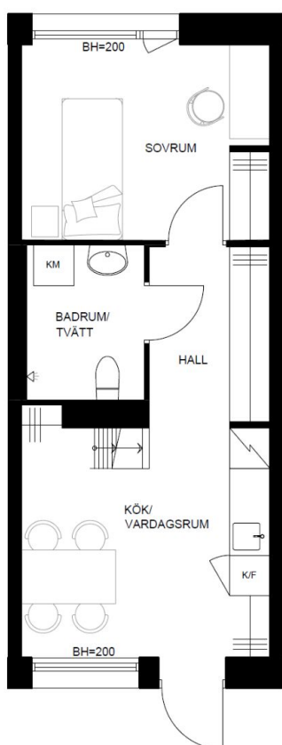
NEDRE PLAN
