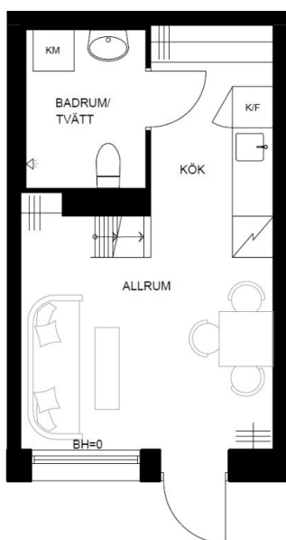
NEDRE PLAN
