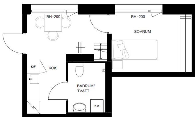
NEDRE PLAN
